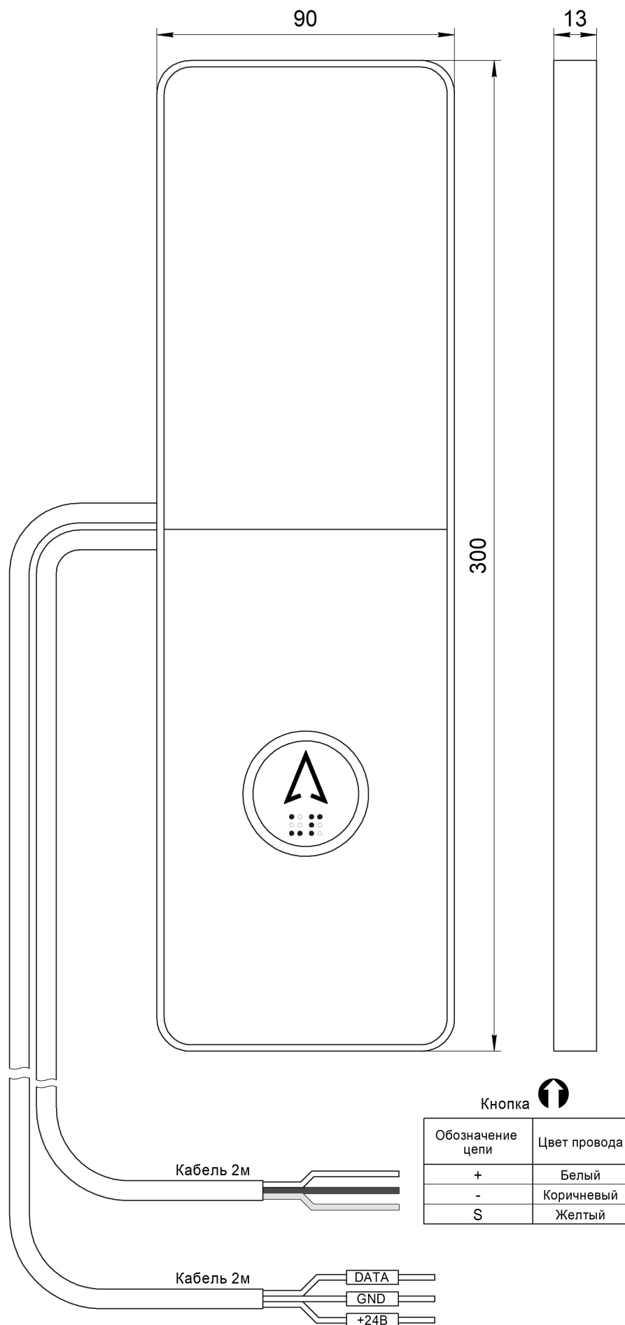
Рис.1 Внешний вид Вызывной пост ОНИКС НШЕК.468381.027
